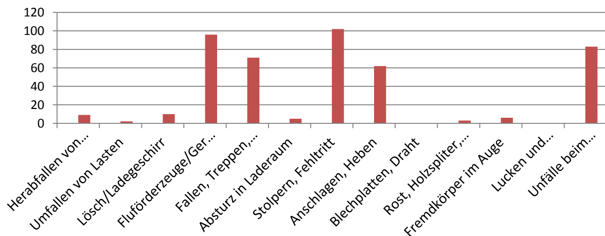
Abb. 32: Unfallursachen
